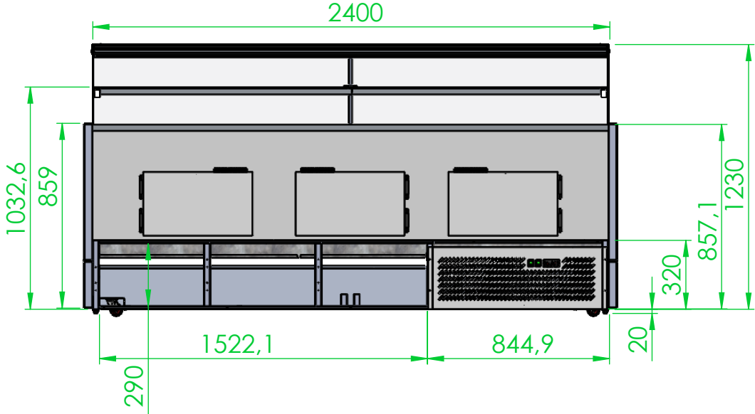
VISTA RETRO (LATO OPERATORE)
